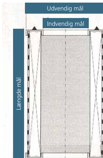
Patron måleskitsetegning
